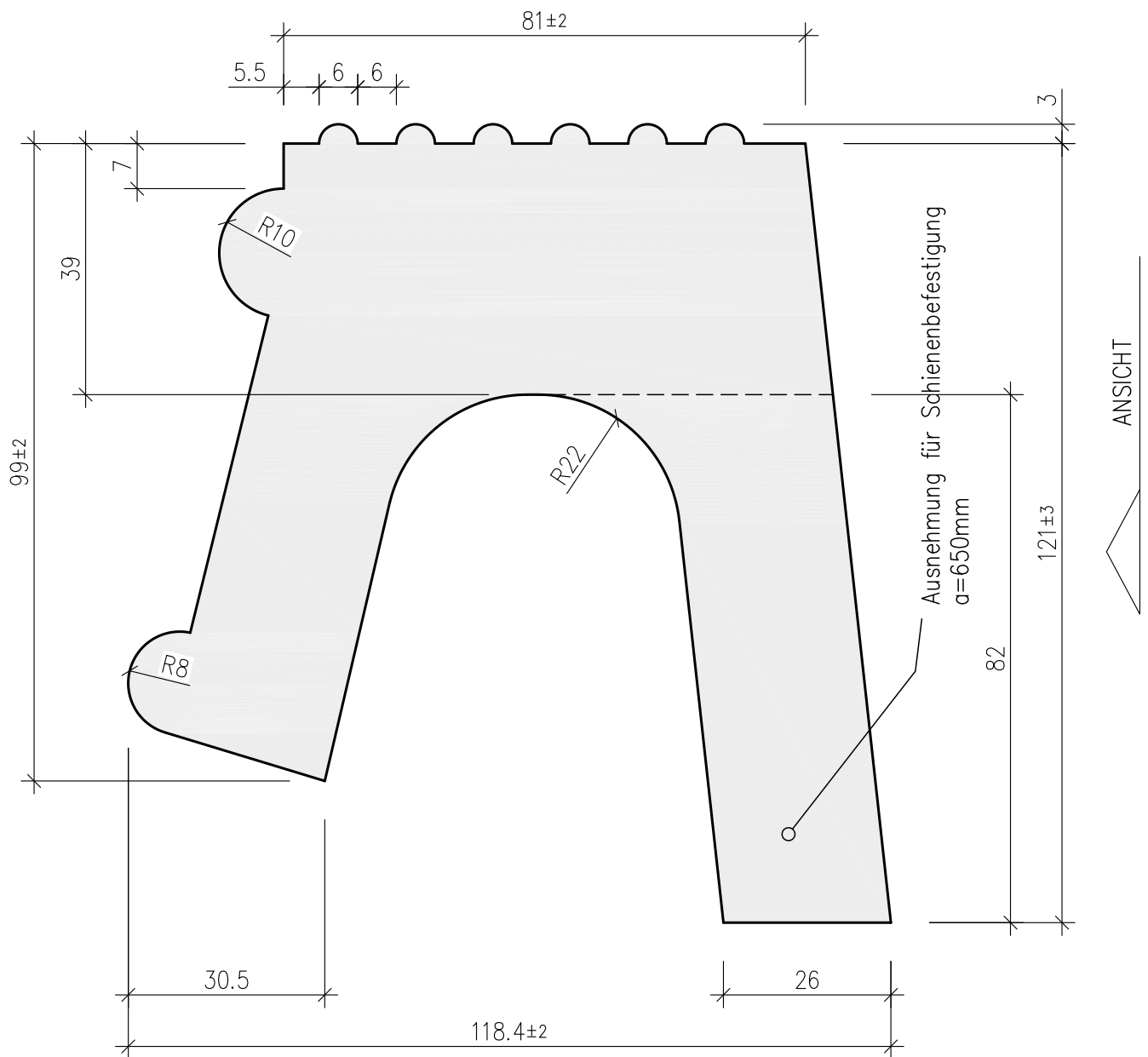
Ansicht 1:10
